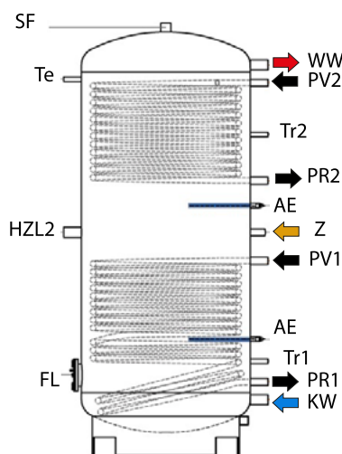
ISSWW 1500÷2000 L
