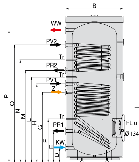
ISSWW 200÷500
